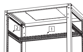
1. Belka montażowa CLASSIC 2. Belka poprzeczna CLASSIC
