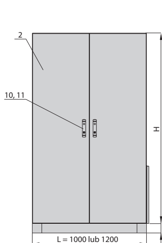
Widok z przodu (szafa dwudrzwiowa)
