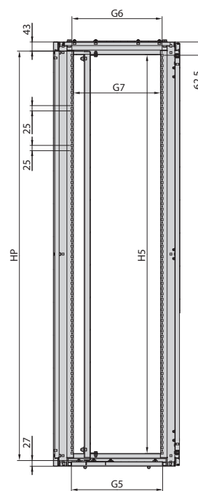
Przekrój A-A
