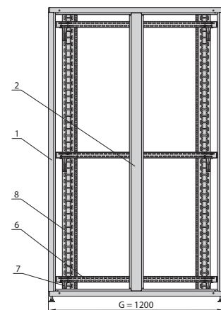
Widok z boku (szafa o głębokości 1200 mm)
