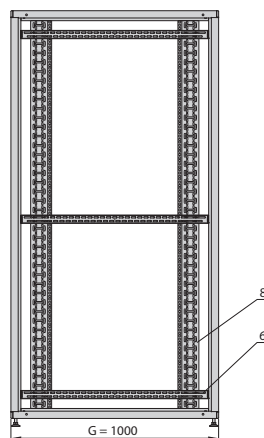
Widok z boku (szafa o głębokości 1000 mm)
