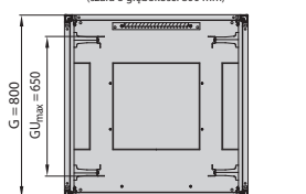
Przekrój D-D (szafa o głębokości 800 mm)
