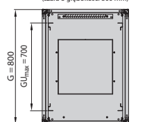
Przekrój C-C (szafa o głębokości 800 mm)
