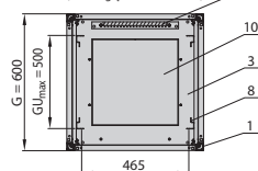
Przekrój C-C (szafa o głębokości 600 mm)
