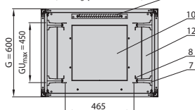
Przekrój D-D (szafa o głębokości 600 mm)
