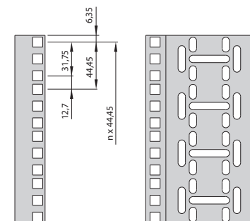
Belka nośna 19" typu PREMIUM, głębokość 12 mm
