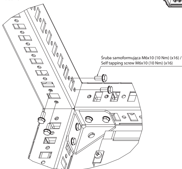
Szczegół C / Detail C
