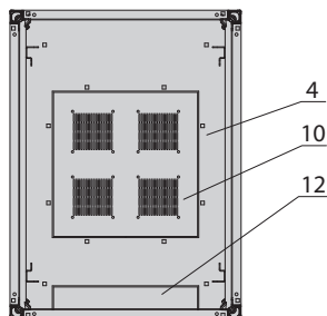
A-A section
