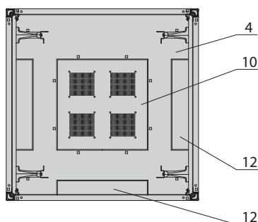
A-A section
