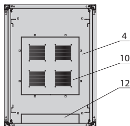
A-A section
