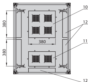
A-A section
