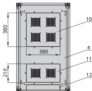
A-A section
