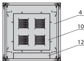
A-A section
