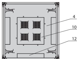
A-A section
