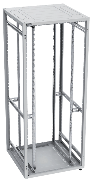
Szafa o szerokości 800 mm z zestawem wzmacniającym Dopuszczalne obciążenie 1500 kg
