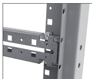
Ceownik bez klamry
