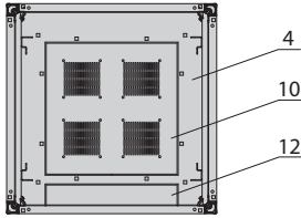
A-A section
